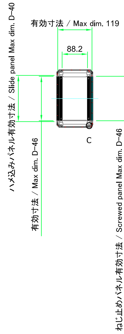
B-B ( 1 : 8 )
